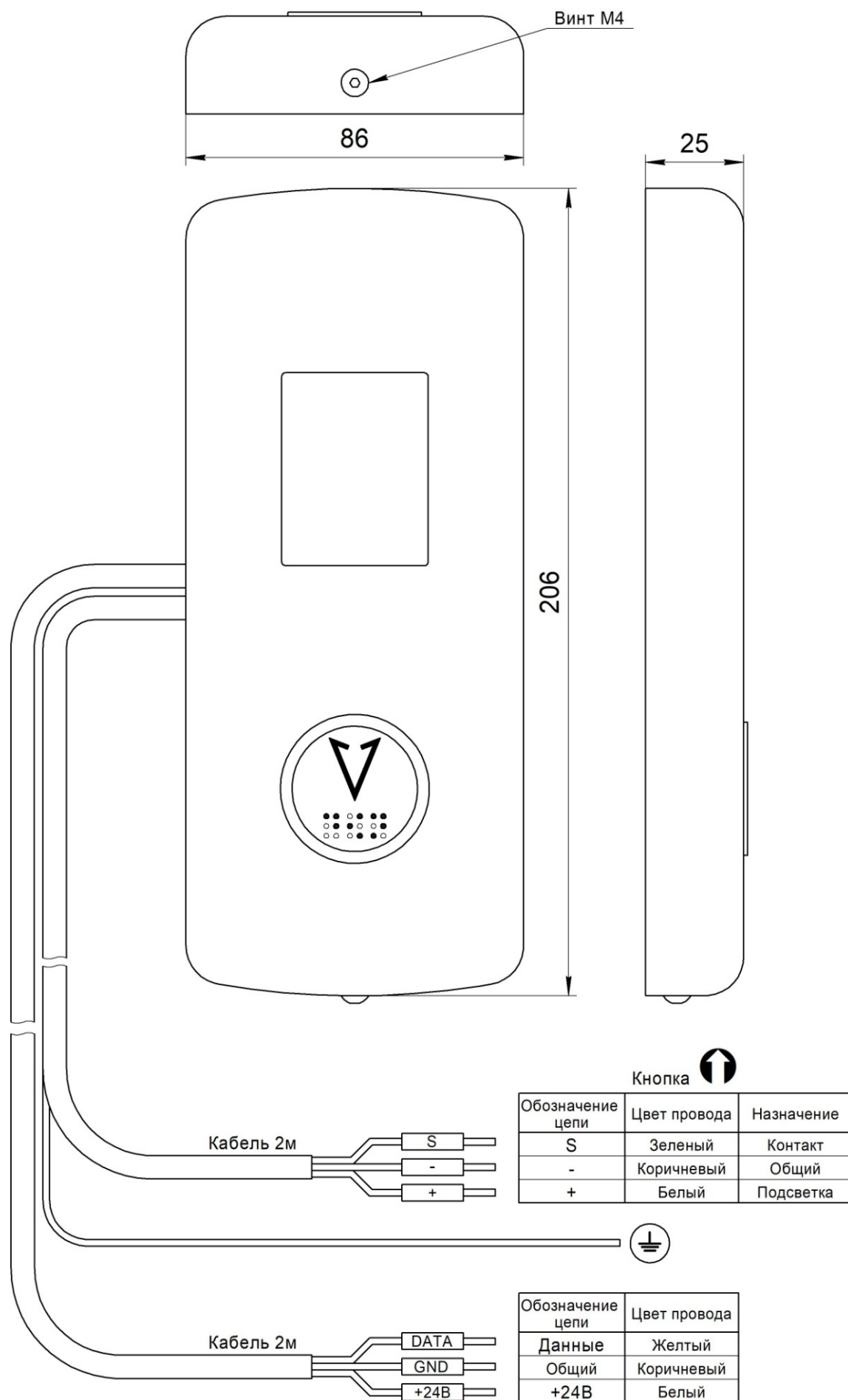
Рис.1 Внешний вид, габаритные и установочные размеры Вызывного поста ВП-1102-1074-07
